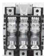
Vista de Cápsulas de vacío S10
